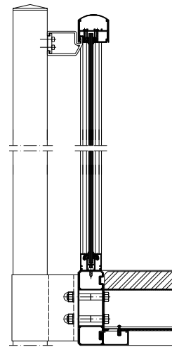
Befestigung auf der Stahlbeton-Balkonplattform Fixing onto the steel-reinforced concrete balcony platform
